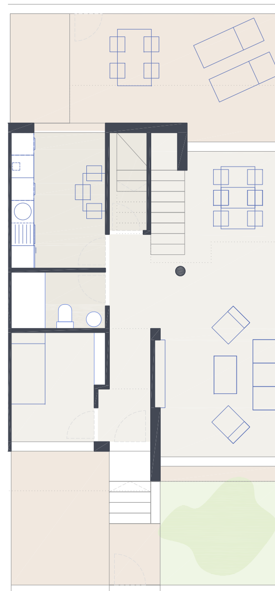
PLANTA BAJA TIPO B
