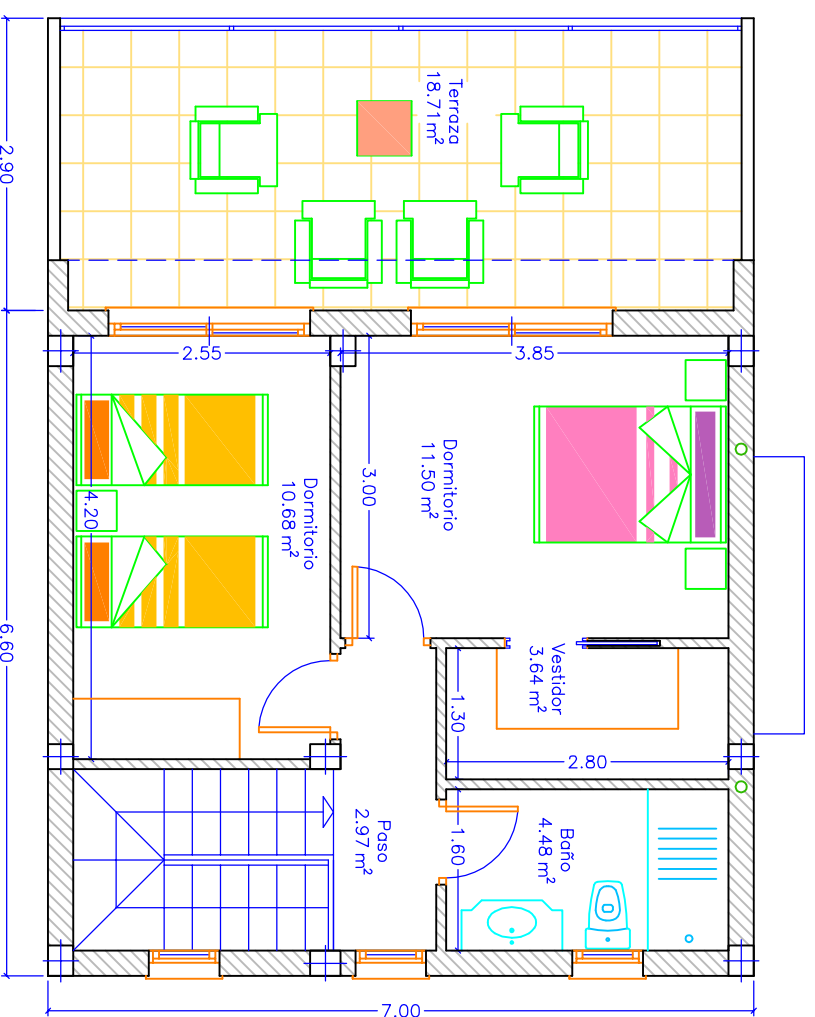
PLANTA 1, S.C. = 46.20 M 2
