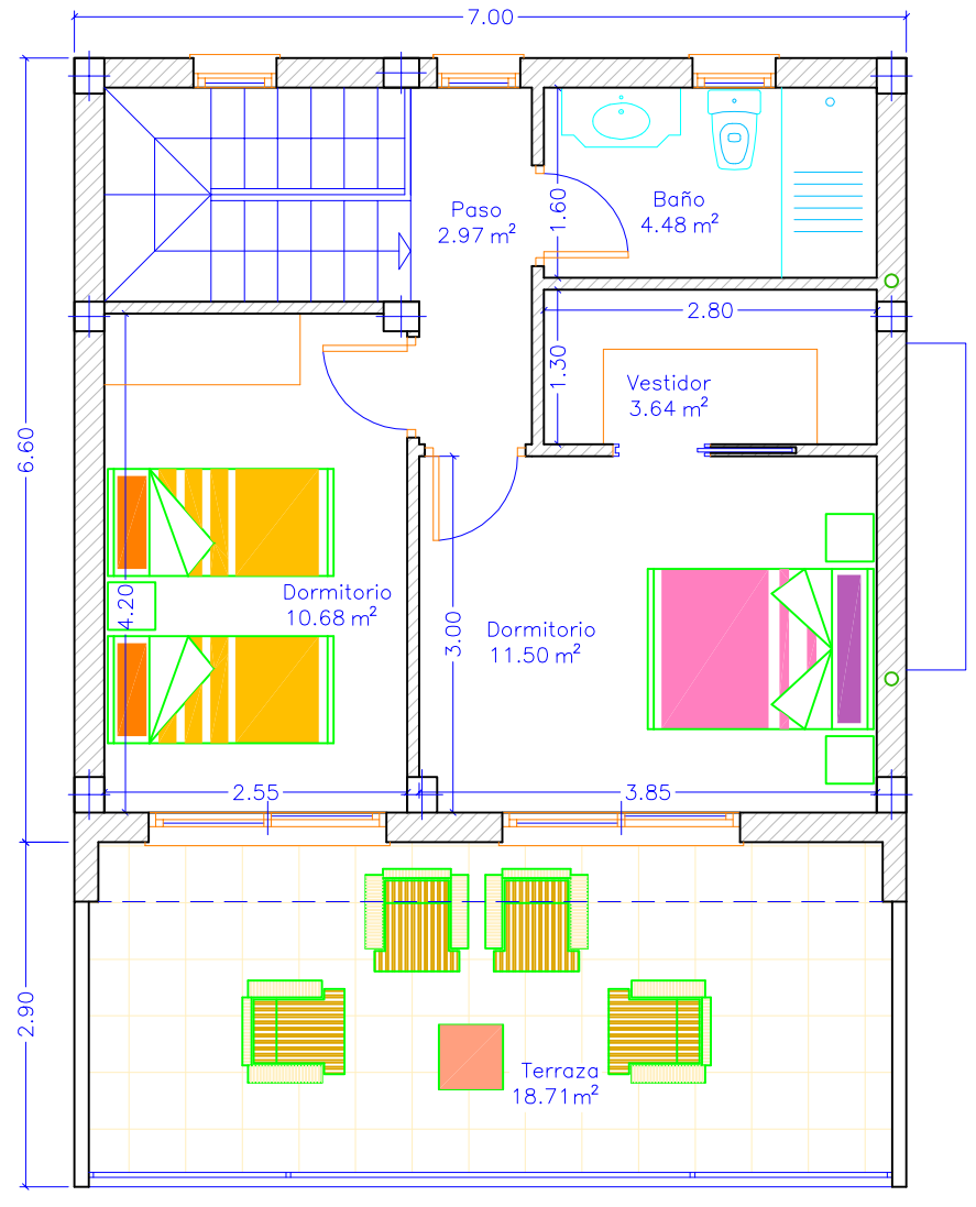
PLANTA 1, S.C.= 46.20 M2
